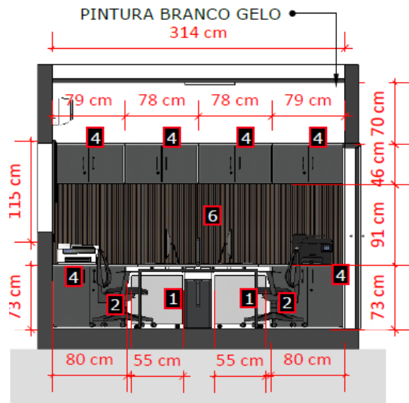
04 VISTA C ESC.: 1/50
