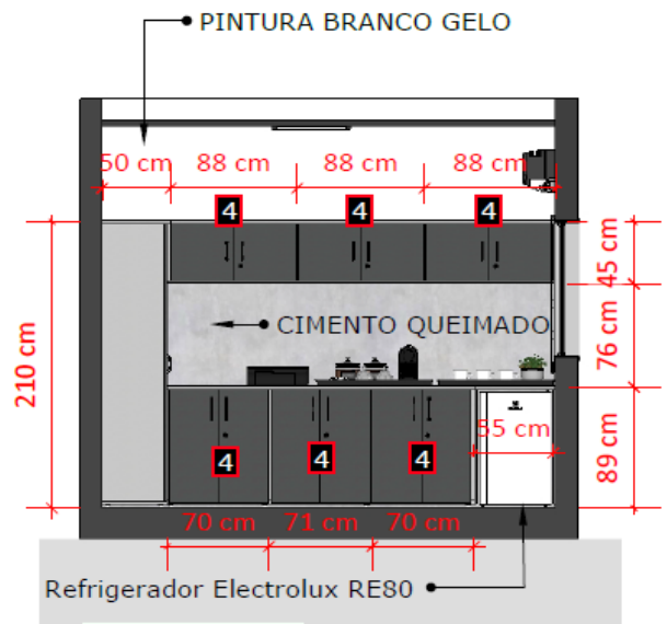
05 VISTA D ESC.: 1/50
