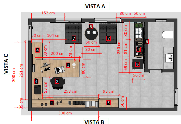
01 PLANTA BAIXA DE LAYOUT ESC.: 1/50
