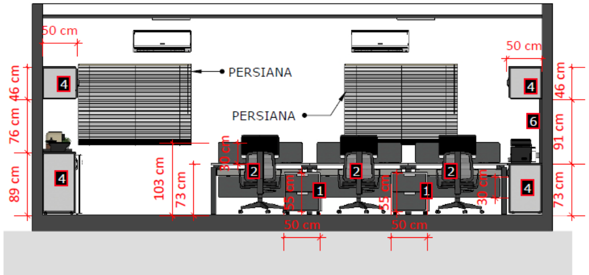
03 VISTA B ESC.: 1/50
