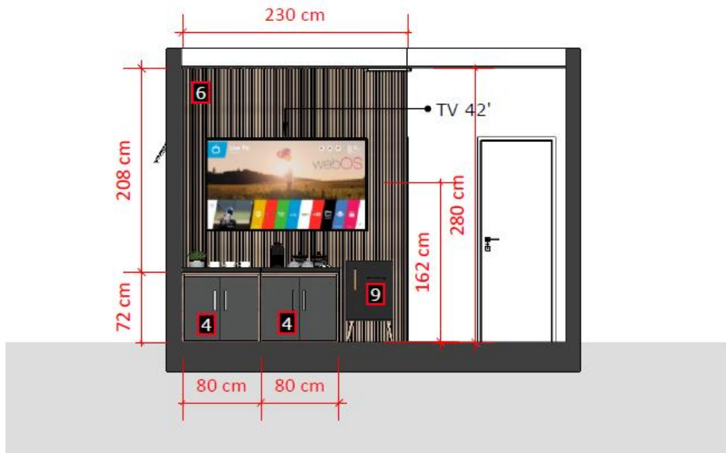
06 VISTA C ESC.: 1/50
