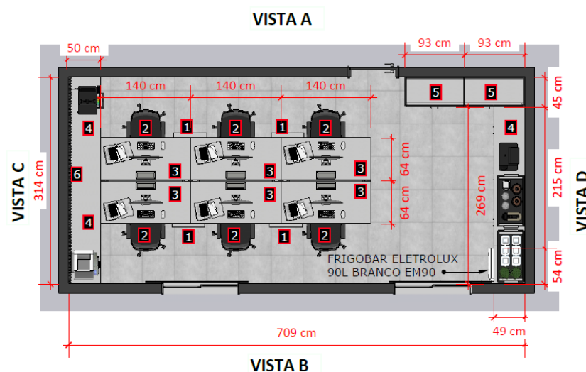
01 PLANTA BAIXA DE LAYOUT ESC.: 1/50
