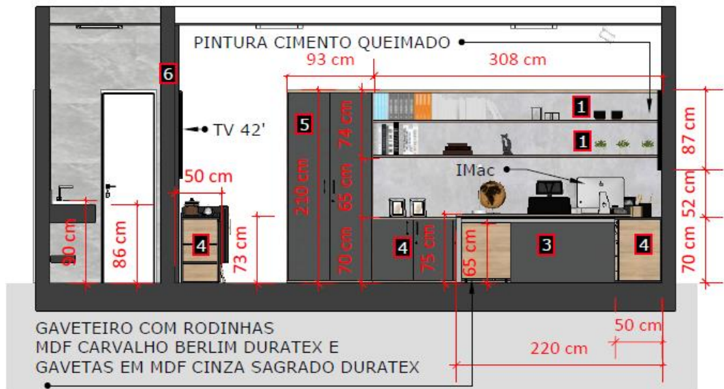
05 VISTA B - RECUADA ESC.: 1/50
